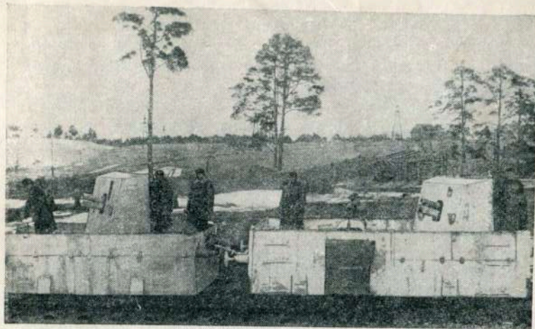
Железнодорожные артиллерийские бронеплощадки, оборонявшие в годы блокады Ленинграда линию между Сестрорецком и Белоостровом.
